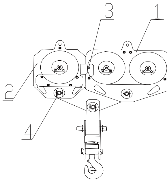
1-主吊钩 2-副吊钩 3-销轴 c 4-销轴 d
