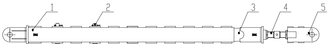
图 4-110 附着撑杆
