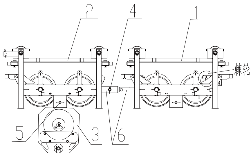
1-主小车 2-副小车 3-副吊钩 4-销轴 a 5-销轴 b 6-连接座 a
