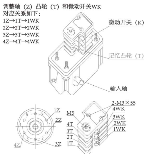
图 4-95 起升限位器图
