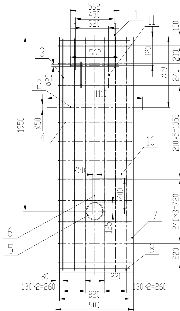
图 3-9 2100kg配重规格尺寸图
