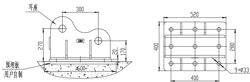
图 4-112 耳座
