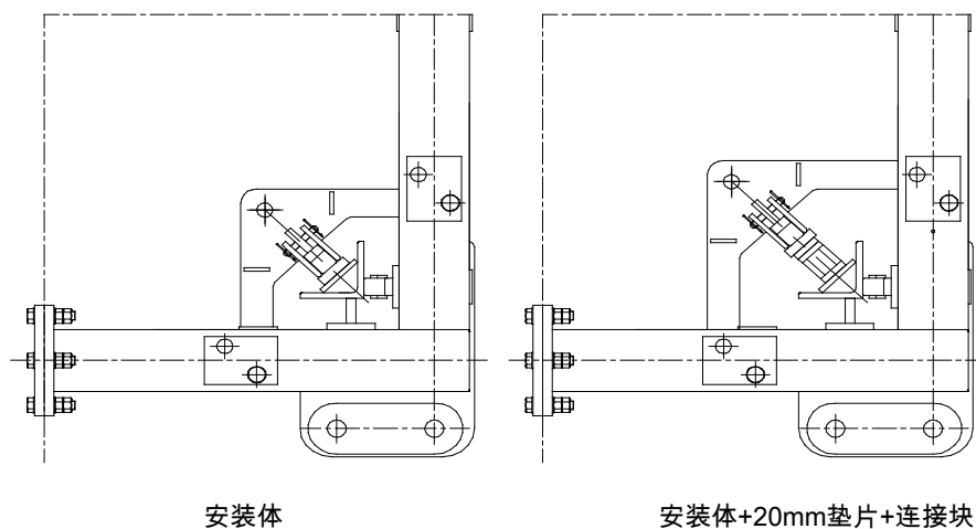
图 4-119 有踏步筋板位置安装组合方式
