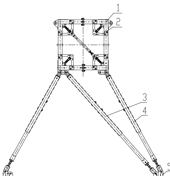
图 4-109 附着架
