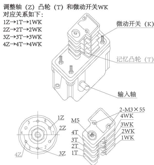
图 4-97 变幅限位器图
