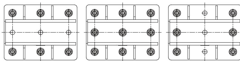
图 4-113 螺栓布置图
