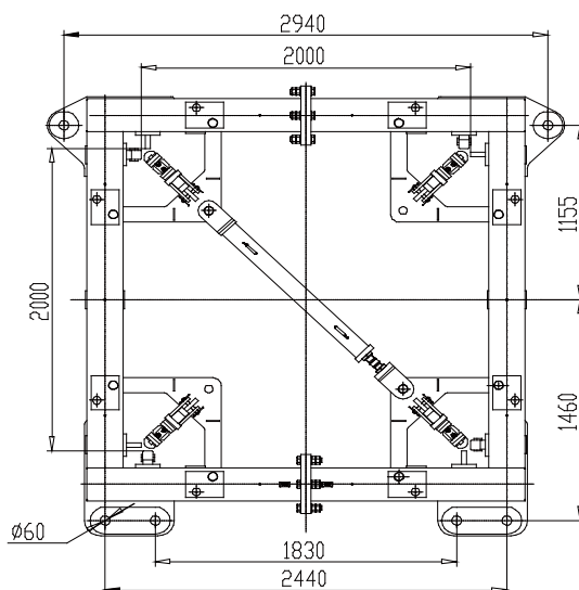
图 4-111 附着框
