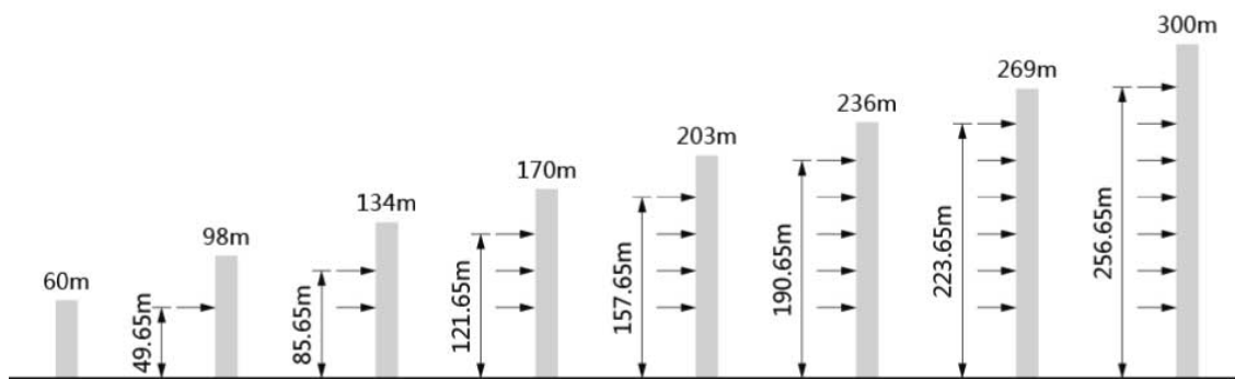
图 4-124 独立固定式及附着架最经济配置示意图
