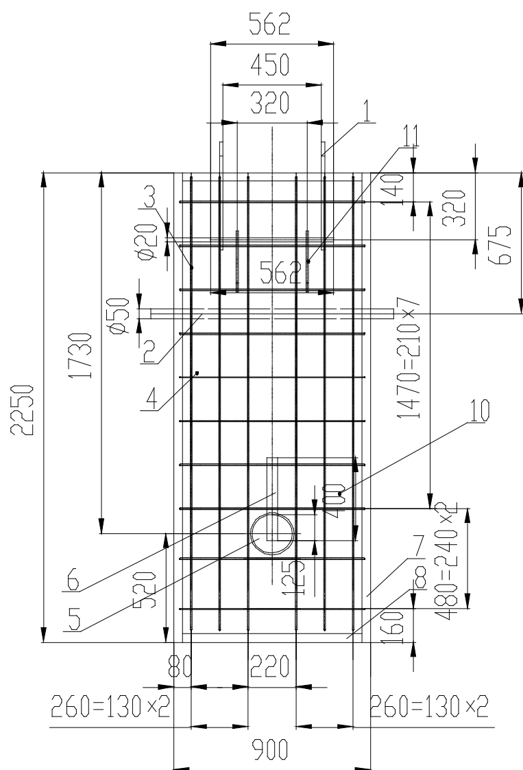
图 3-10 1800kg配重规格尺寸图
