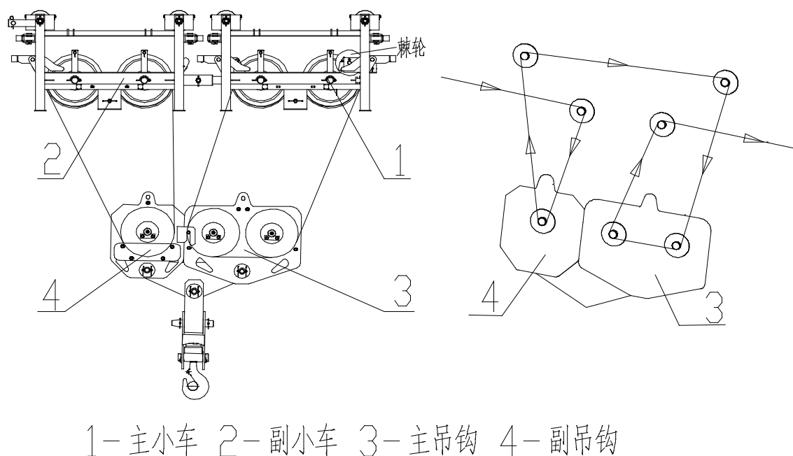
图 4-84 安装和绕绳示意图
