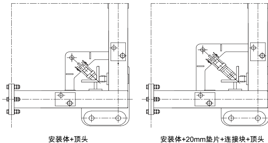
图 4-120 无踏步筋板位置安装组合方式
