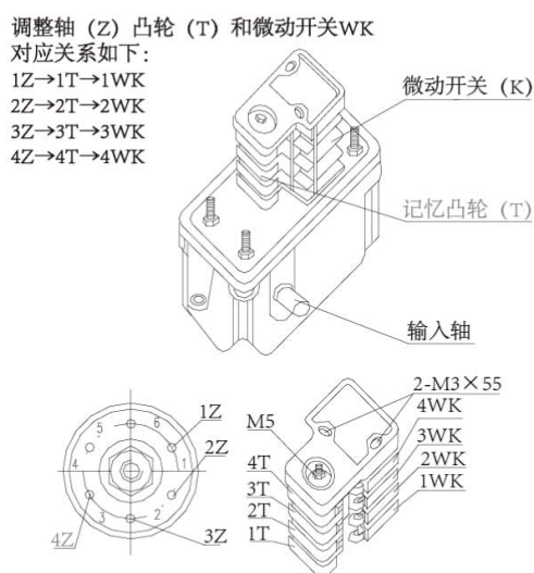
图 4-96 回转限位器图
