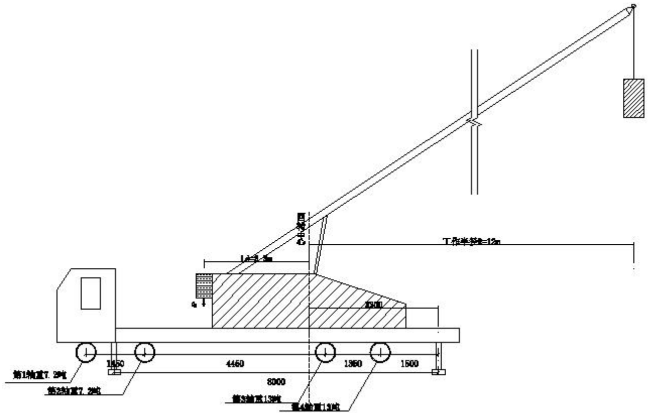
支腿力计算简图
