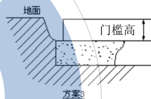
图1.2-3 混凝土基础方案3
