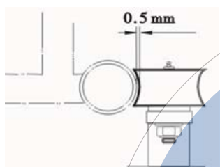
图1.5-1 滚轮间隙调整
