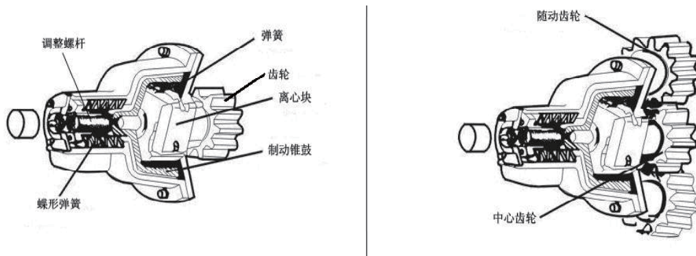
图2.4-1 防坠安全器
