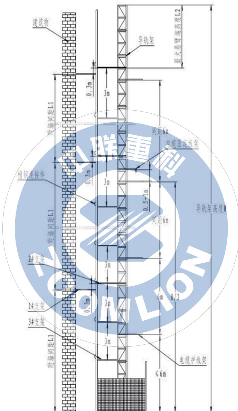
图3.4-2 III型附墙架及电缆护线架安装示意图
