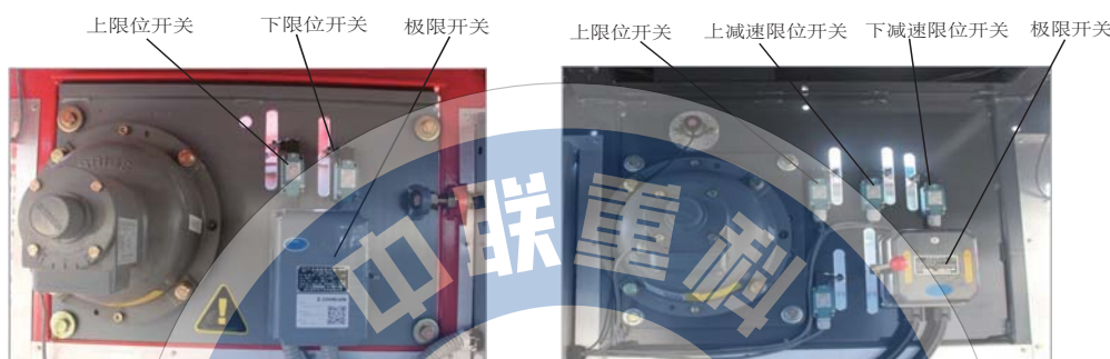
图2.5-1 限位装置
