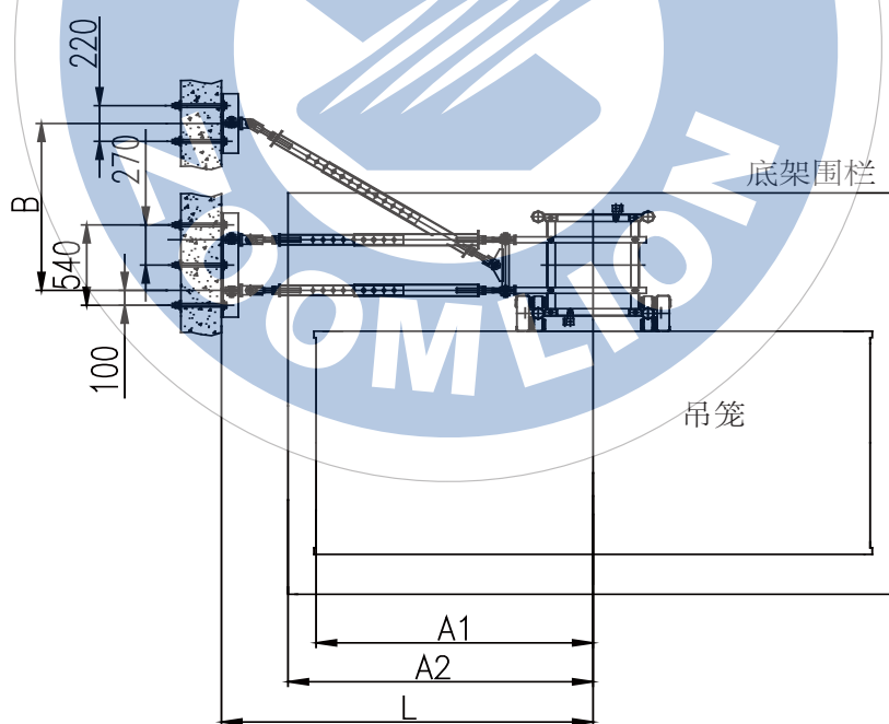
图3.2-1 Ⅰ型附墙架示意图
