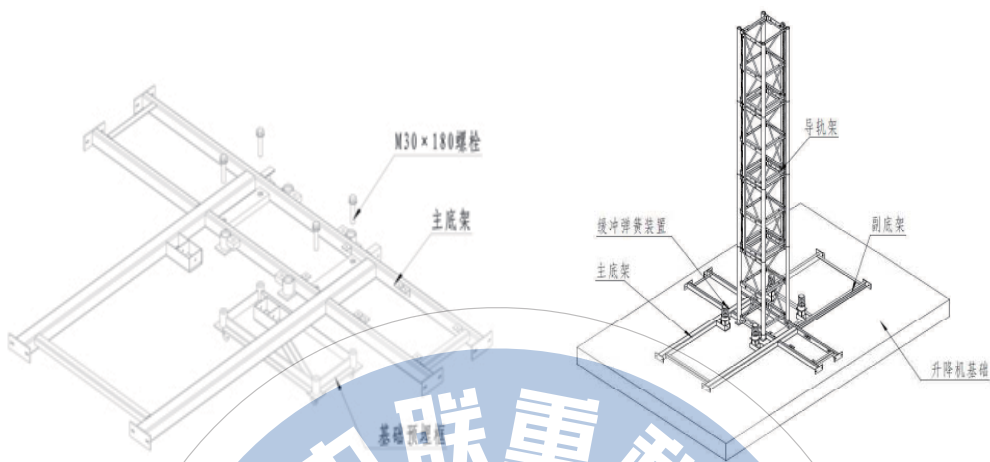
图1.3-3 底架安装图
