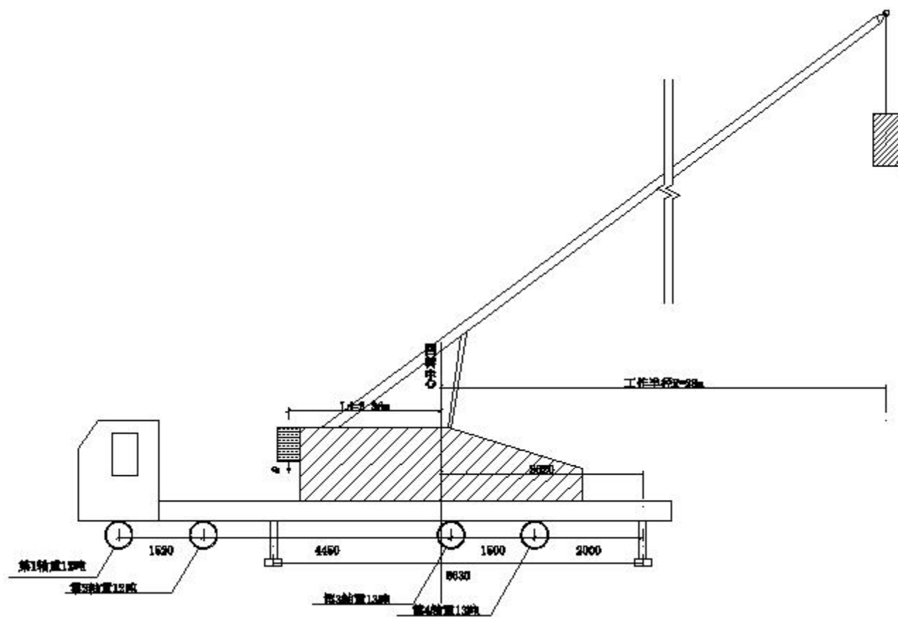
支腿力计算简图
