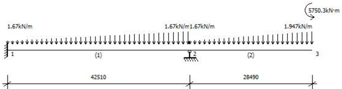
计算简图
