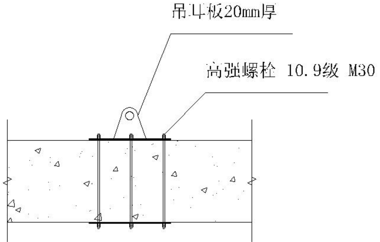
塔机附着节点详图-单吊耳板
