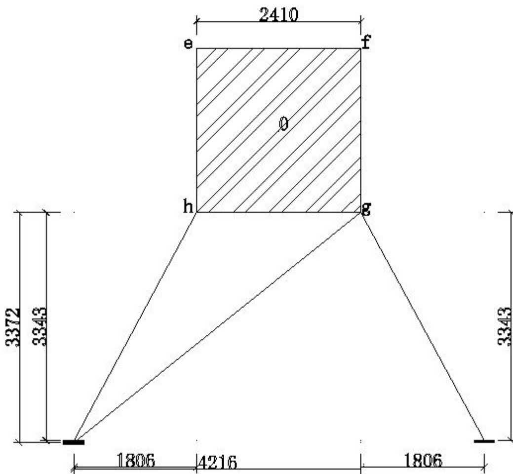
塔机附着平面图
