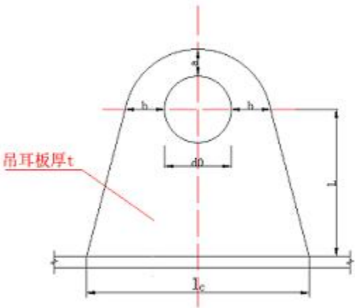
单吊耳板
