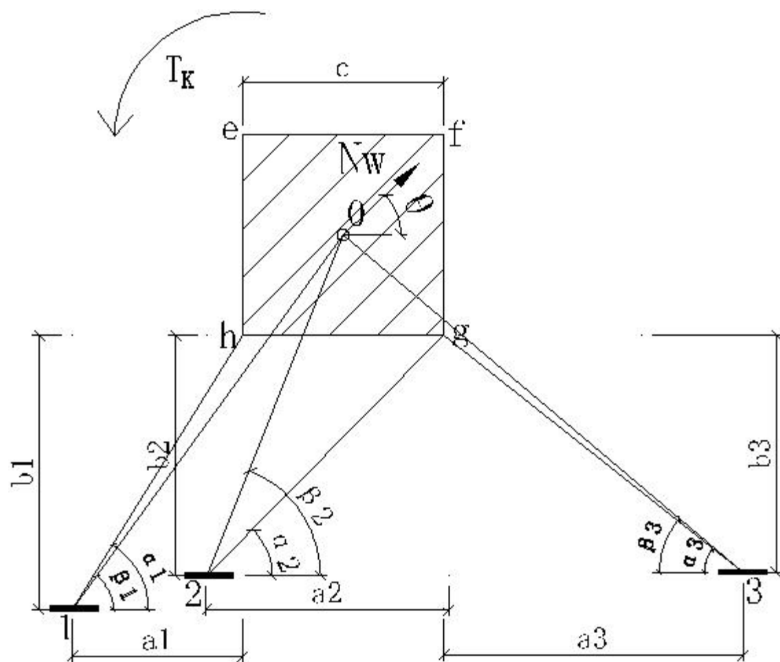
塔机附着示意图
