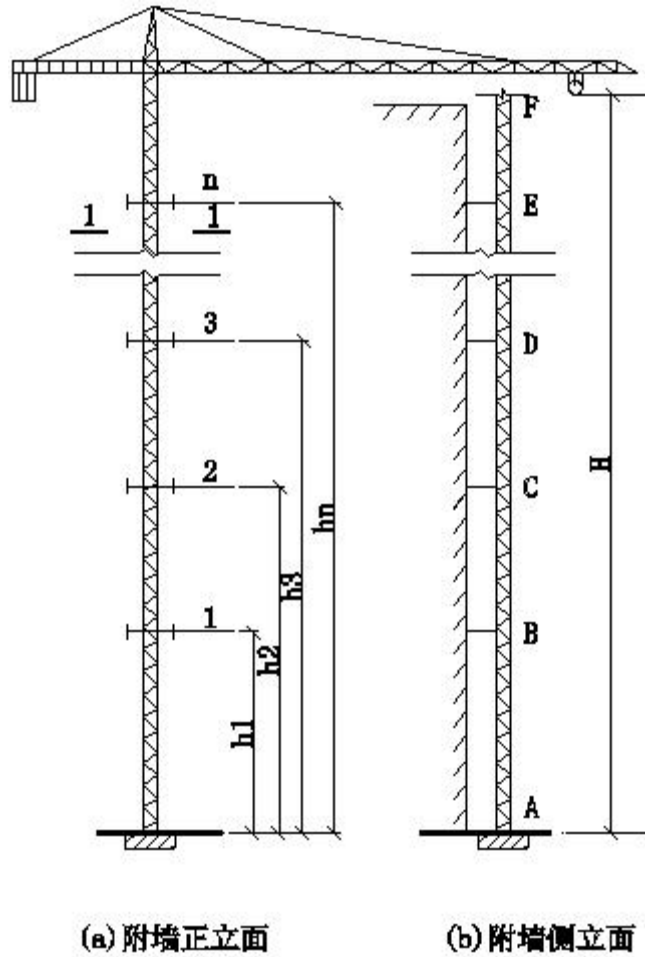
塔机附着立面图
