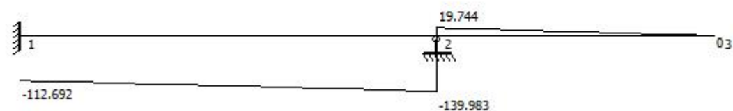
剪力图
