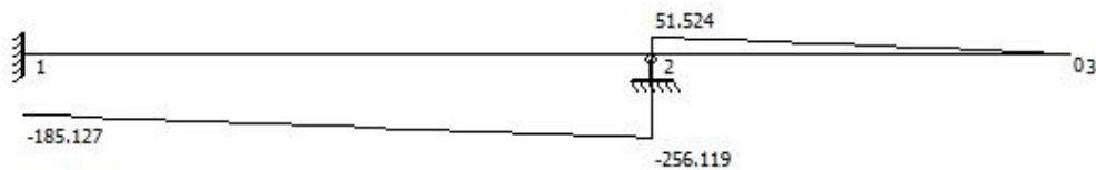
剪力图
