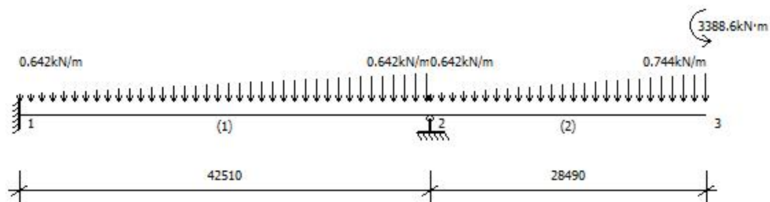
计算简图
